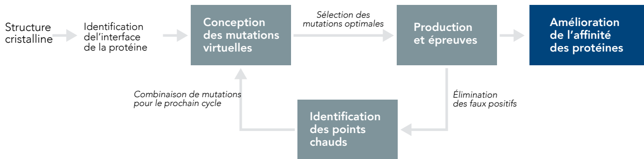
Figure 2 : La plateforme ADAPT comporte une étape automatisée de criblage des mutations. Les prédictions guident la sélection de mutations optimales à l'aide d'une interface web. Les mutants sont ensuite produits afin d'éliminer les faux positifs virtuels et d'identifier les points chauds. La combinaison de points chauds lors des cycles subséquents d'ADAPT mènera à l'obtention d'une séquence optimale.
